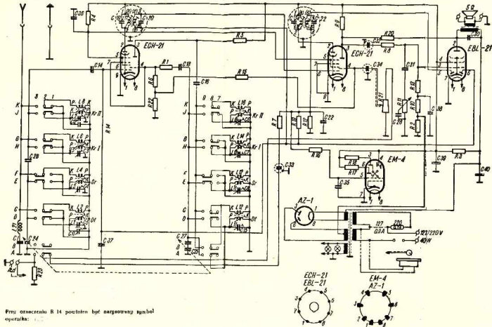
Schemat ideowy odbiornika „Serenada II”
