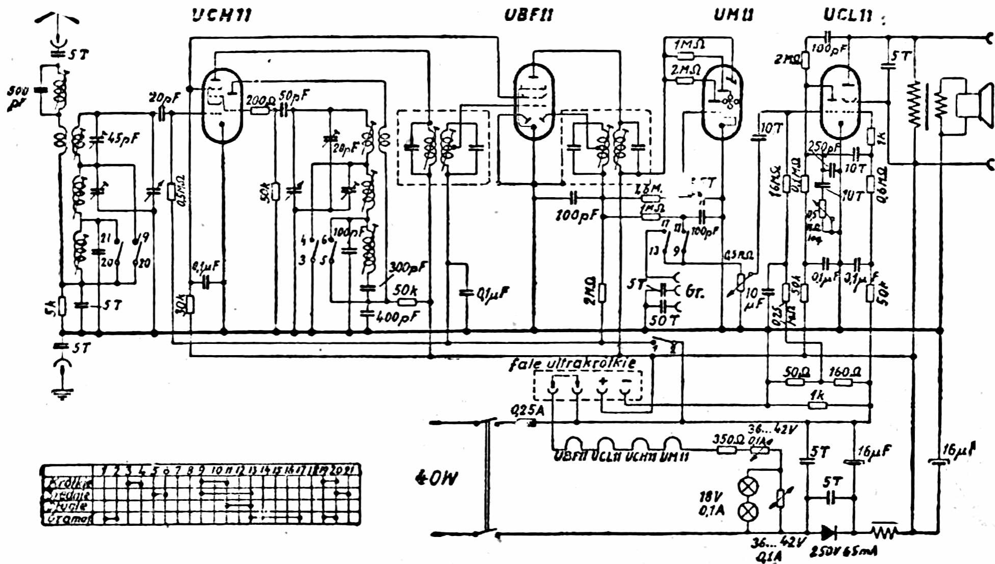
ODBIORNIK R-F-T 5U61
