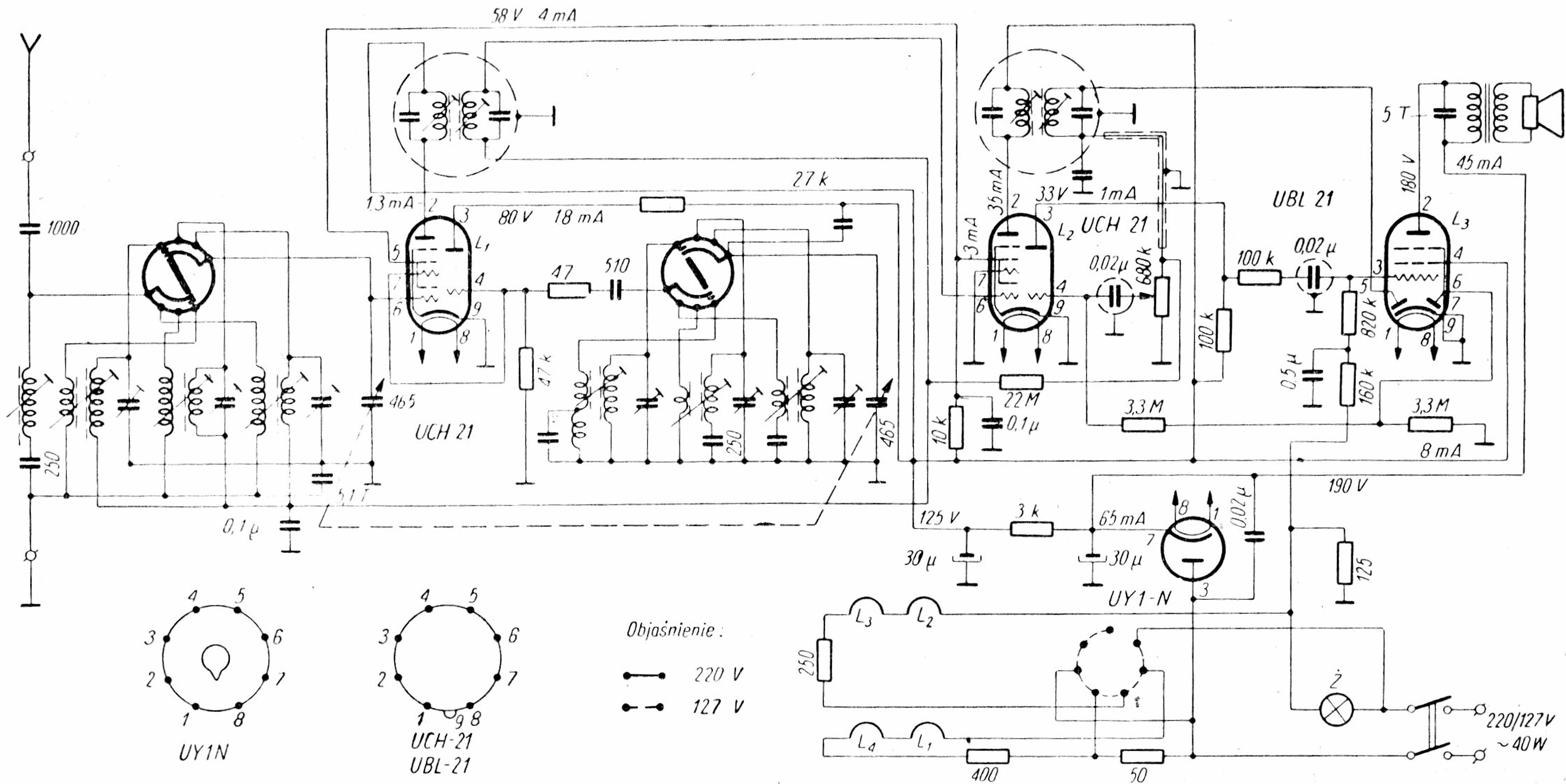
Rys. 1. Schemat ideowy odbiornika „Promyk“
