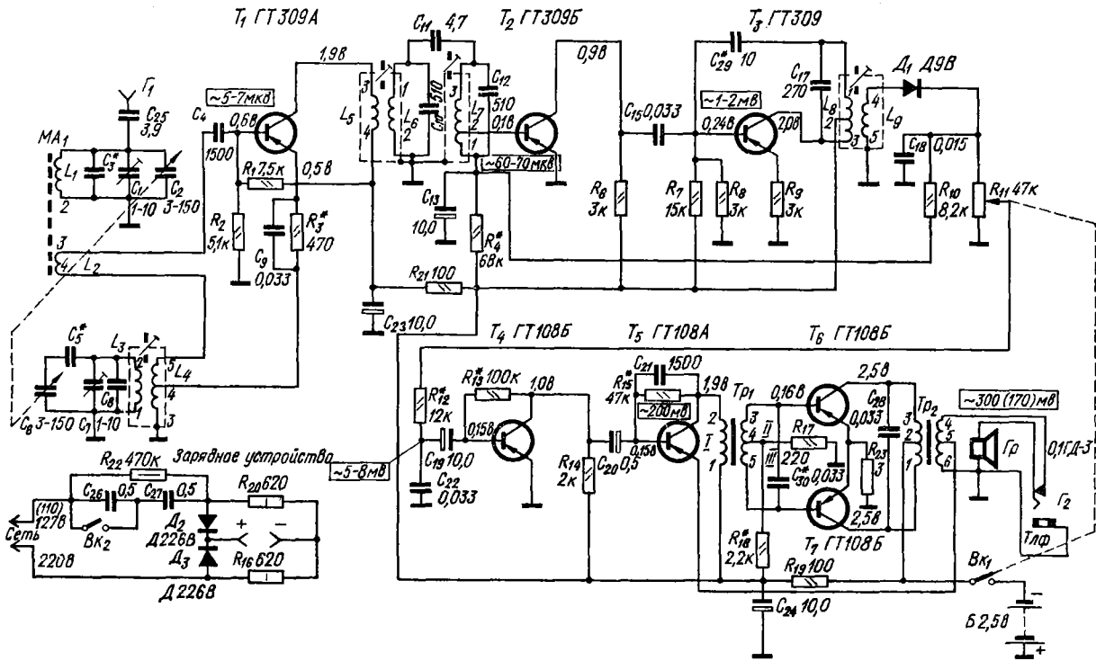
Принципиальная электрическая схема радиоприемников «Космос-М»
