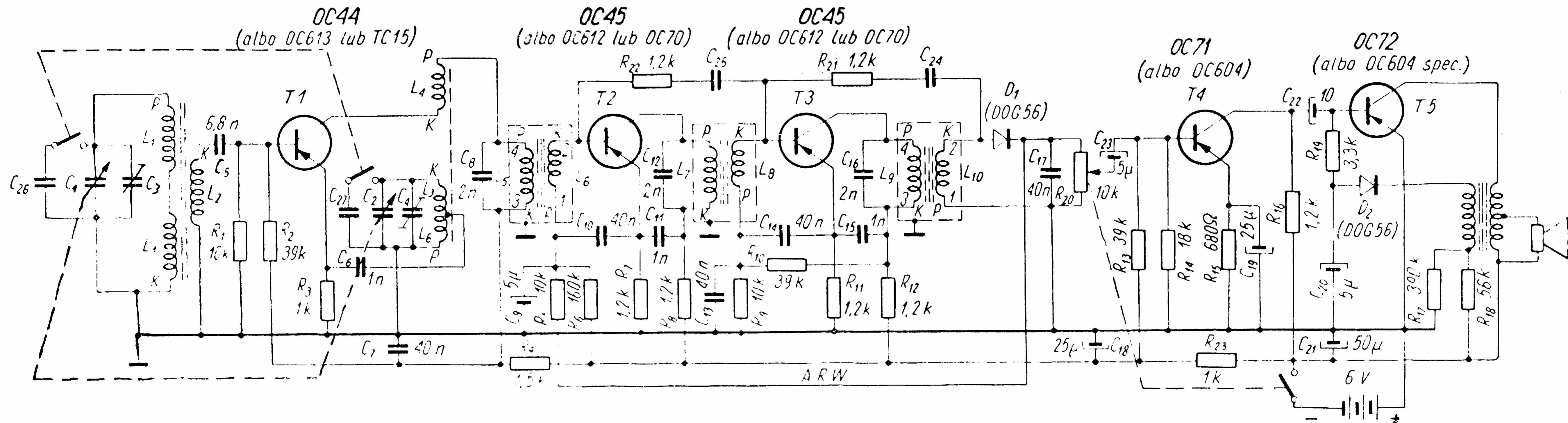
Schemat ideowy odbiornika tranzystorowego „Eltra“
