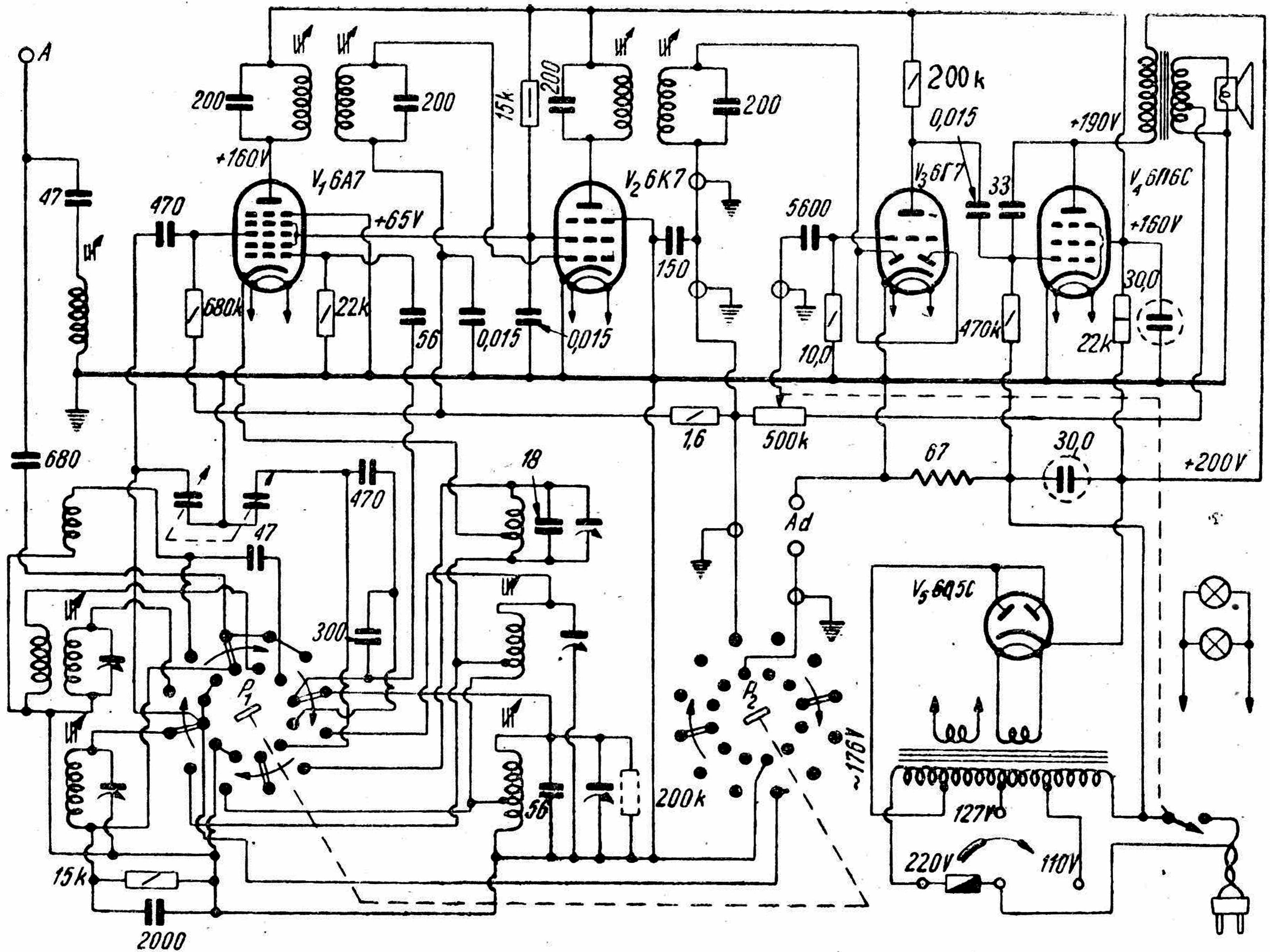
Schemat zasadniczy odbiornika „Dnipro—52“. Oznaczenia lamp na schemacie są podane według nomenklatury radzieckiej. Odpowiednikami lamp są: V_1 — 6SA7, V_2 — 6K7, V_3 — 6SQ7, V_4 — 6V6 i V_5 — 6Z5S
