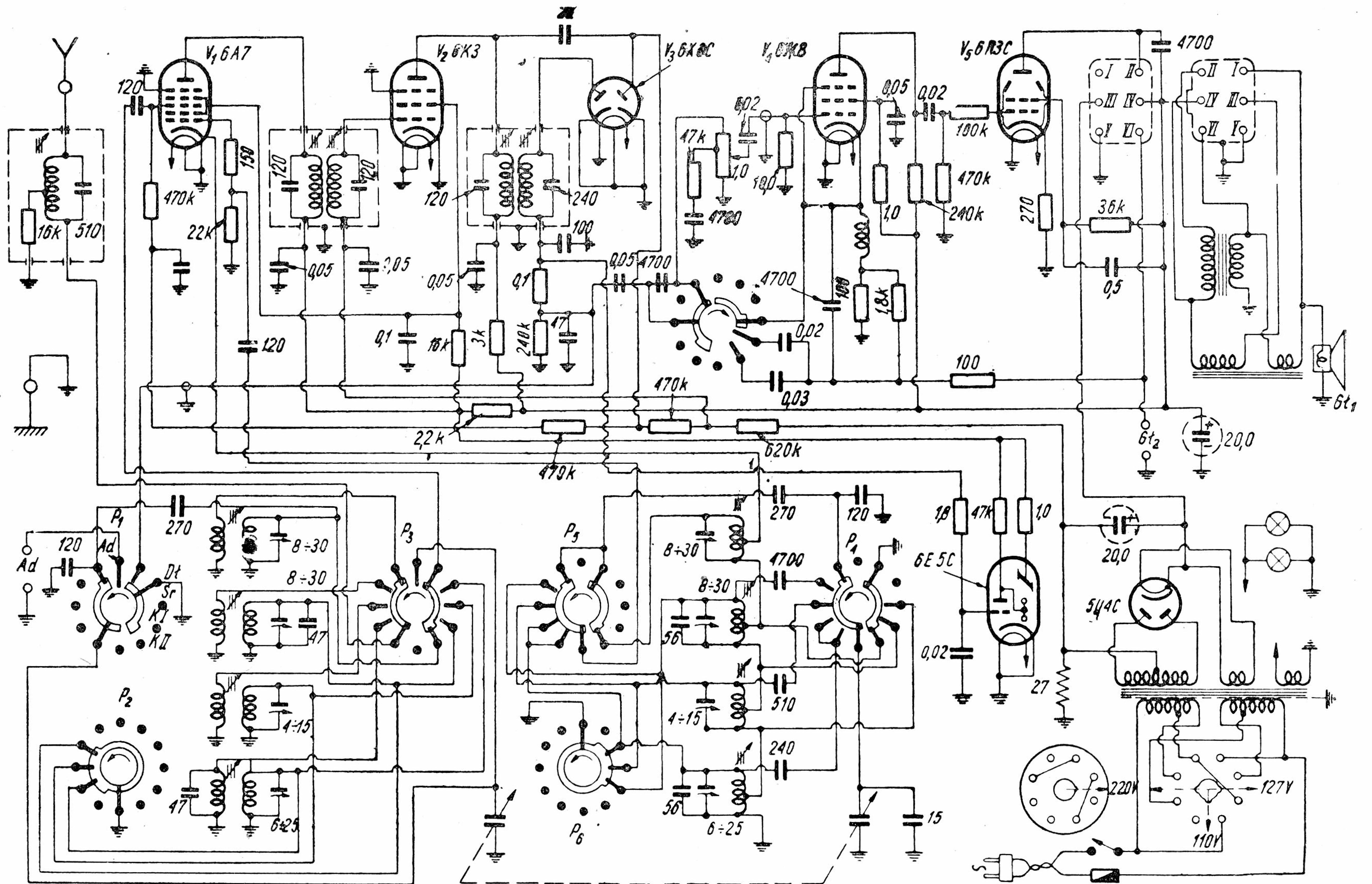
Schemat zasadniczy odbiornika „Baltika“. Oznaczenia lamp na schemacie są podane według nomenklatury radzieckiej. Odpowiednikami lamp są: V_1 — 6SA7, V_2 — 6SK7, V_3 — 6H6S, V_4 — 6SJ7, V_5 — 6P3S, V_6 — 6E5 i V_7 — 5Z4S.
