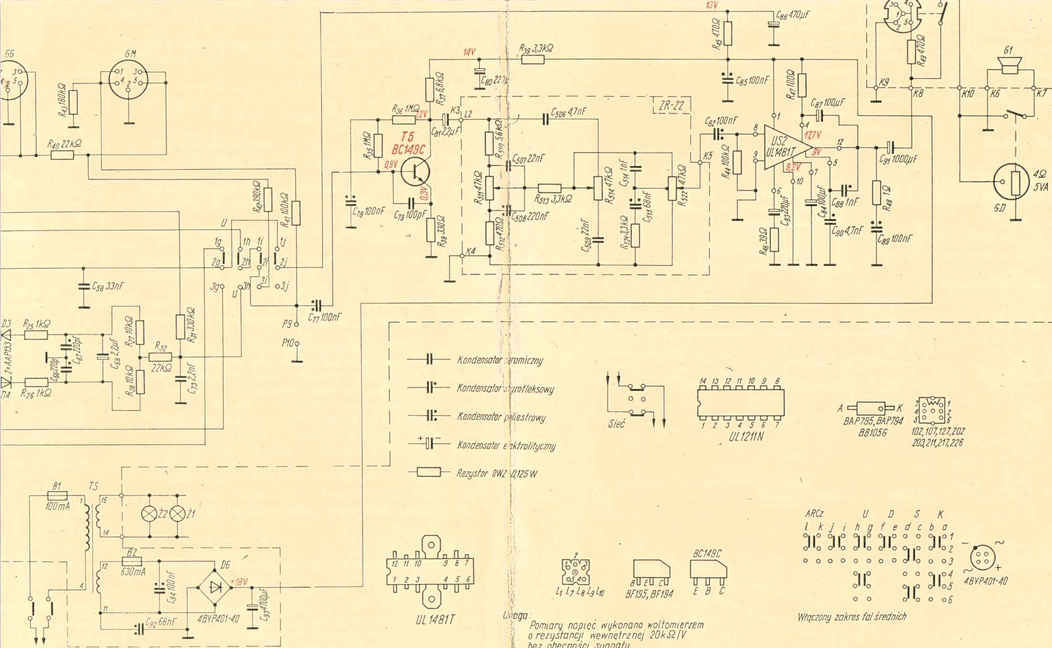
Schemat ideowy odbiornika radiowego „Akord” DMP-501
