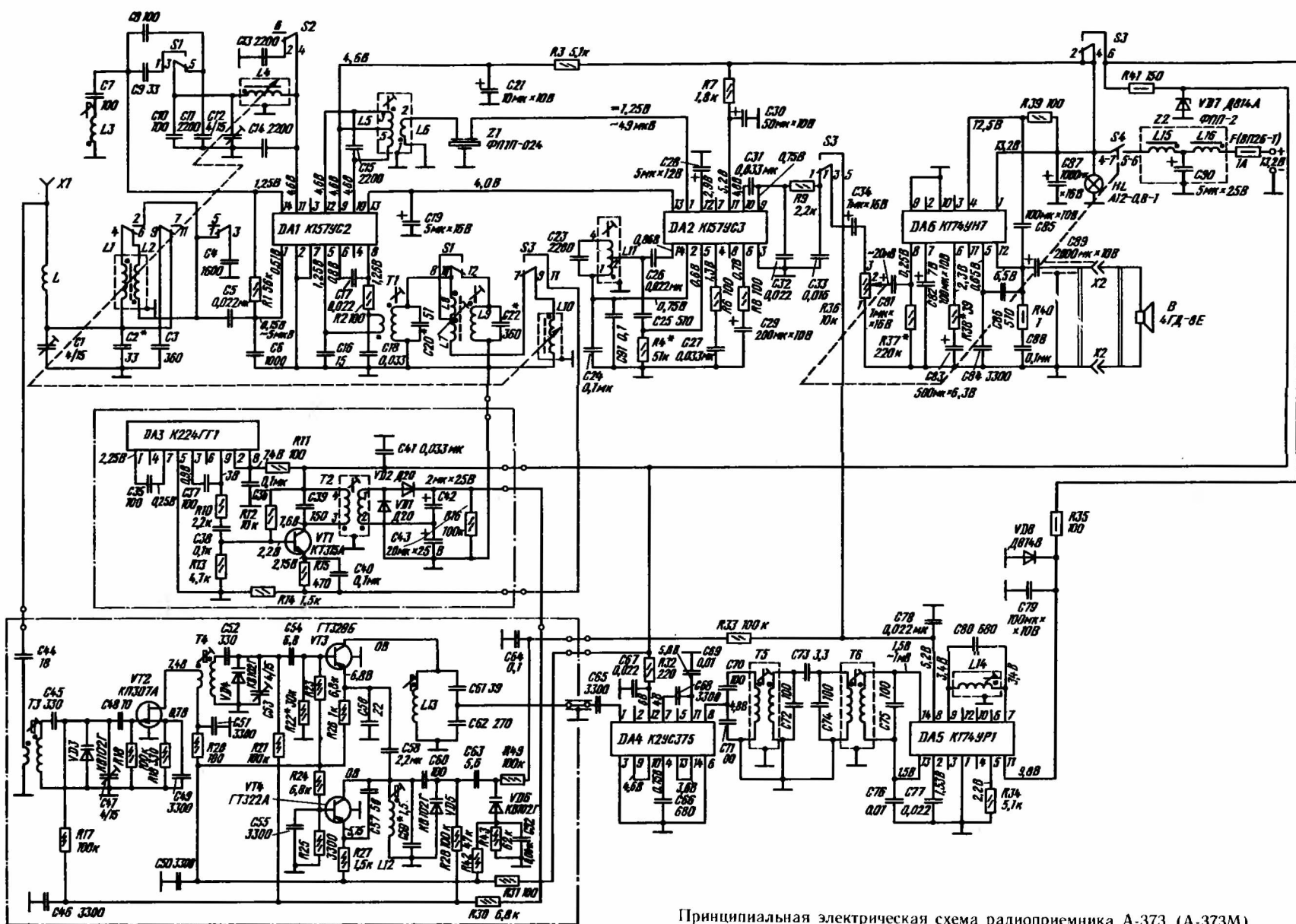
Принципиальная электрическая схема радиоприемника А-373 (А-373М)
