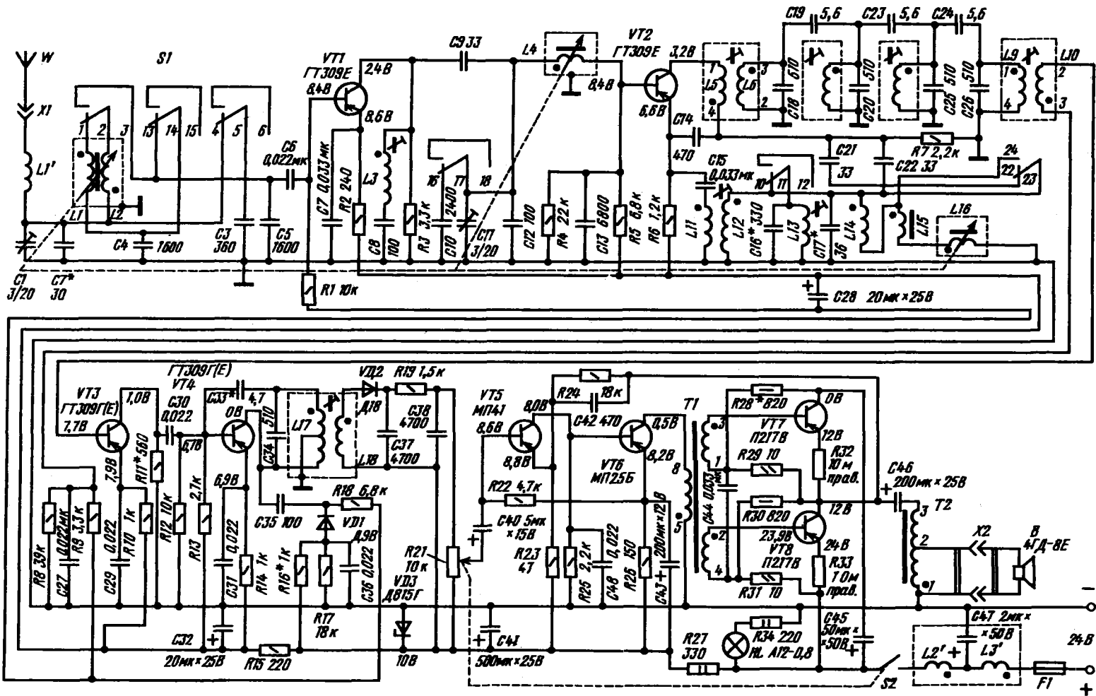
Принципиальная электрическая схема радиопремьника А-324
