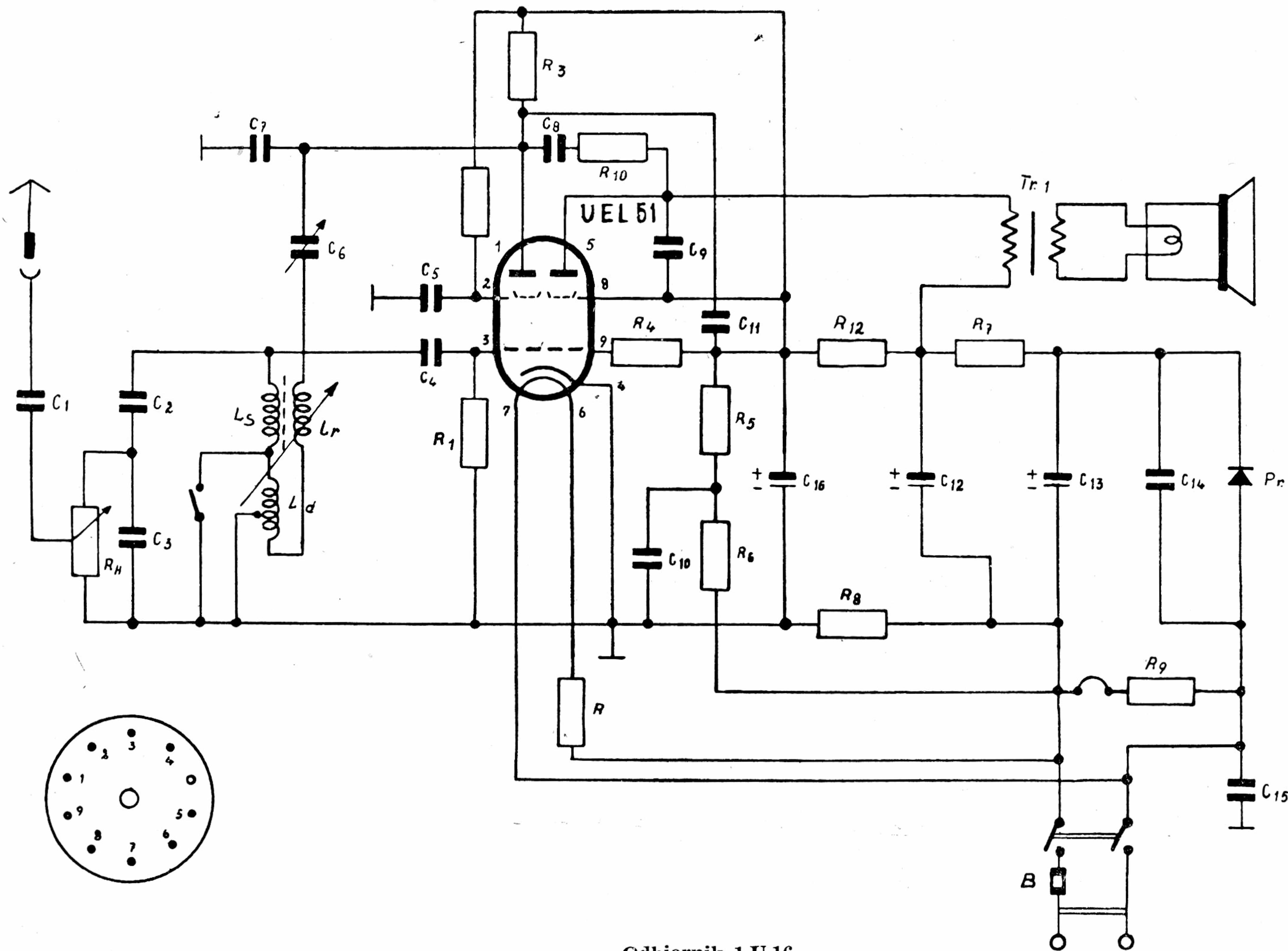
Odbiornik 1 U 16
