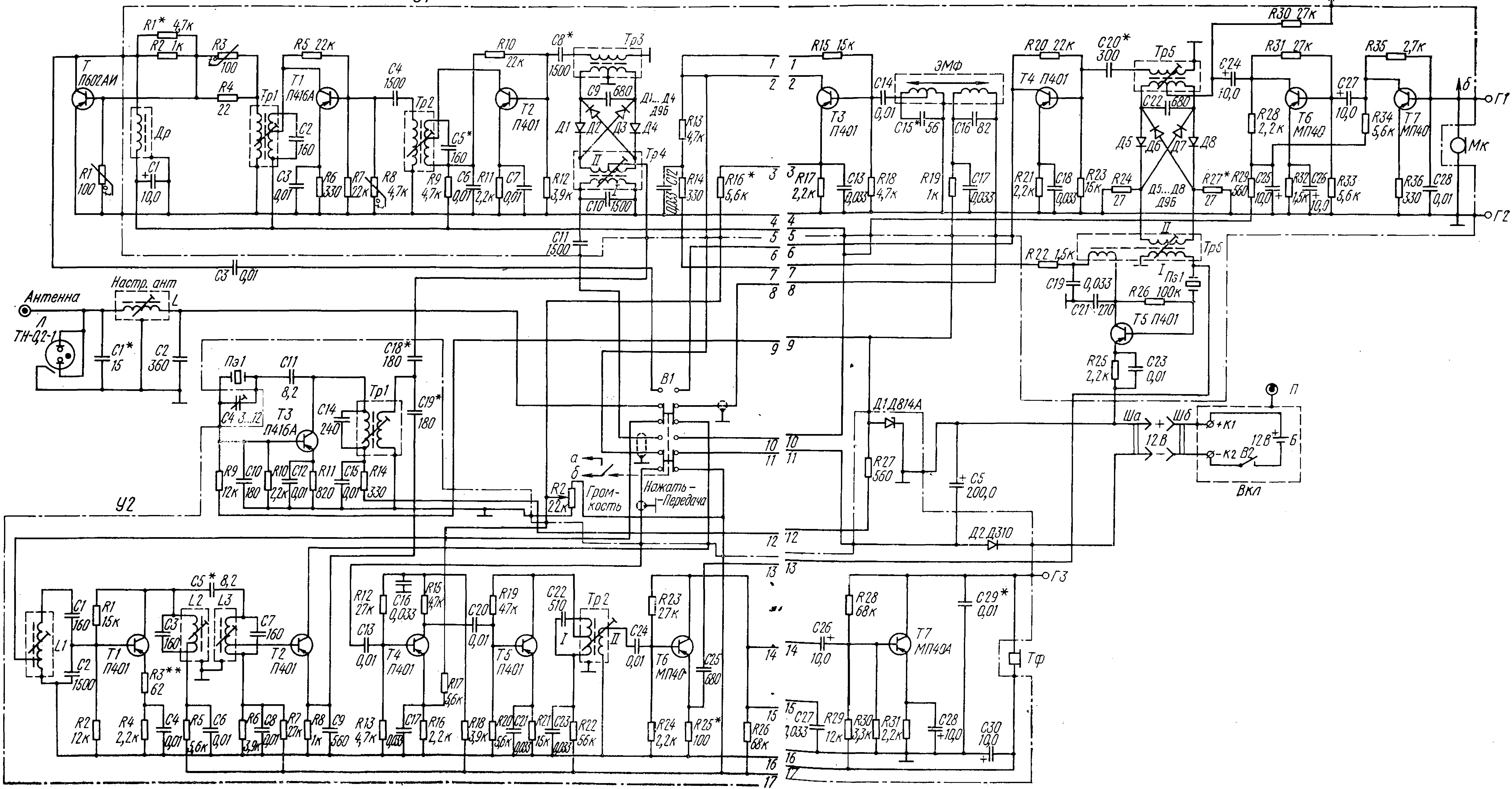
Рис. 2.10. Принципиальная схема радиостанции «Недра-3»
