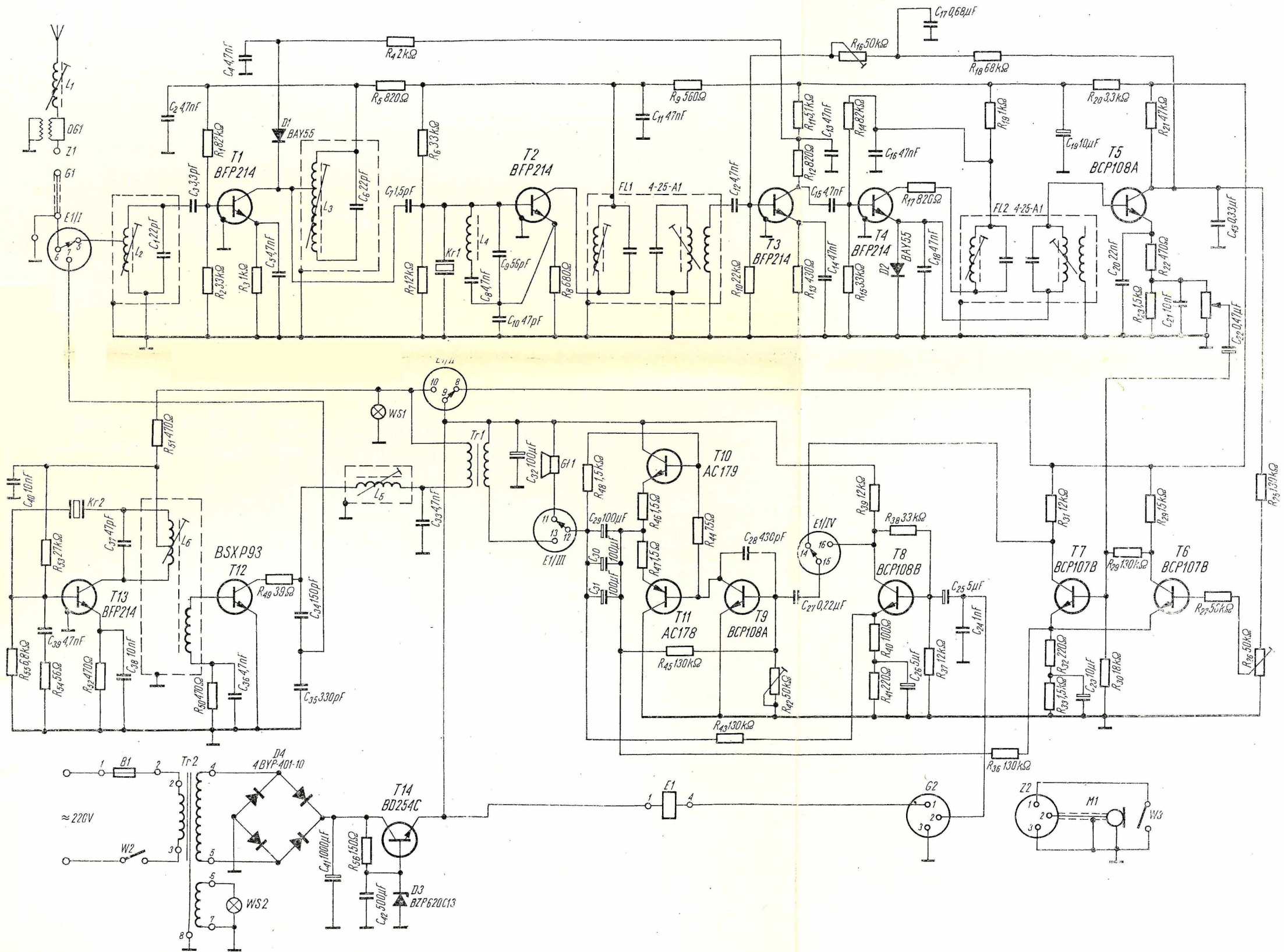
Rys. 8-73. Schemat ideowy zespołu nadawczo-odbiorczego i zasilacza radiotelefonu „Żuraw K”
