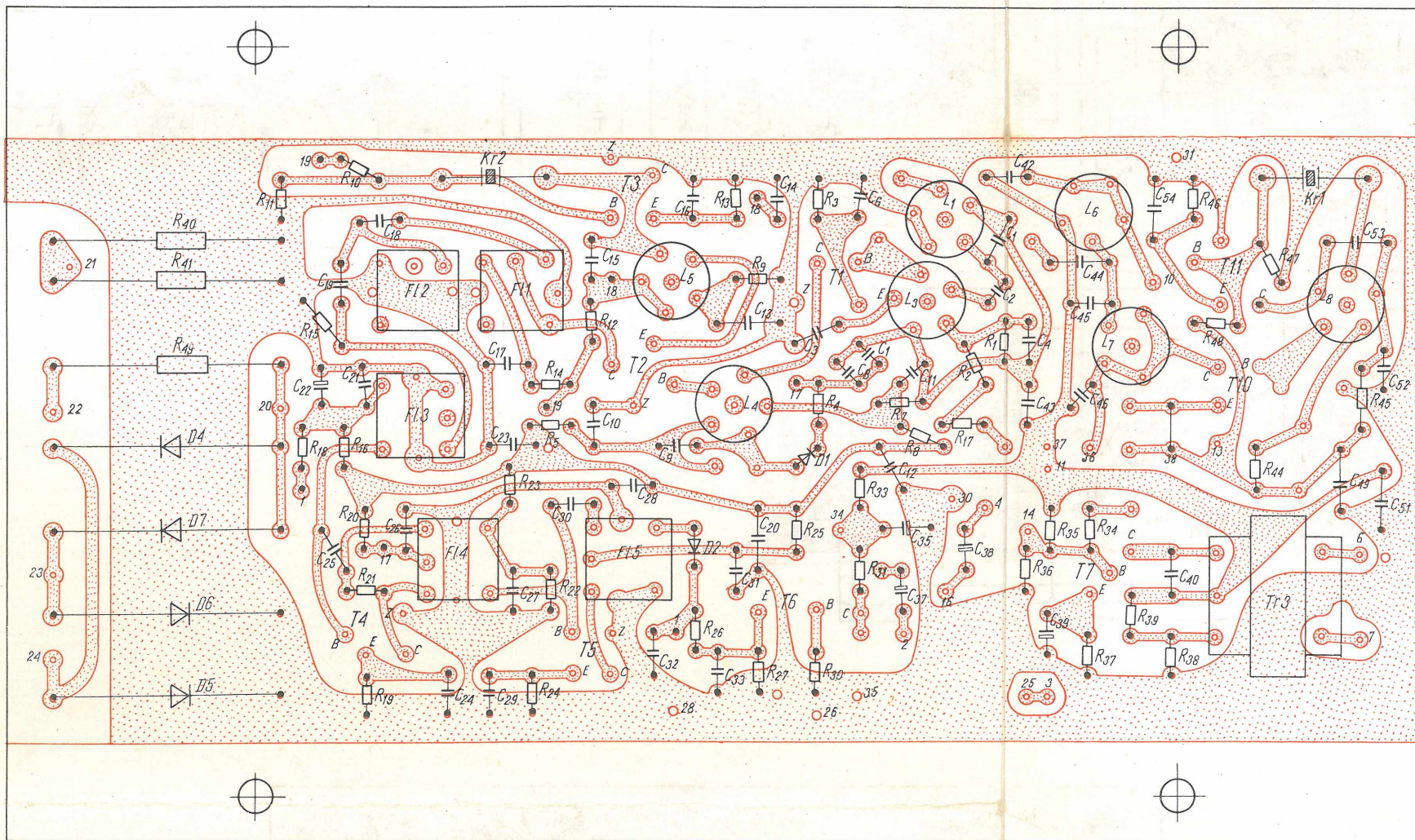
Rys. 8-72. Schemat połączeń drukowanych płytki montażowej radiotelefonu „Żuraw”
