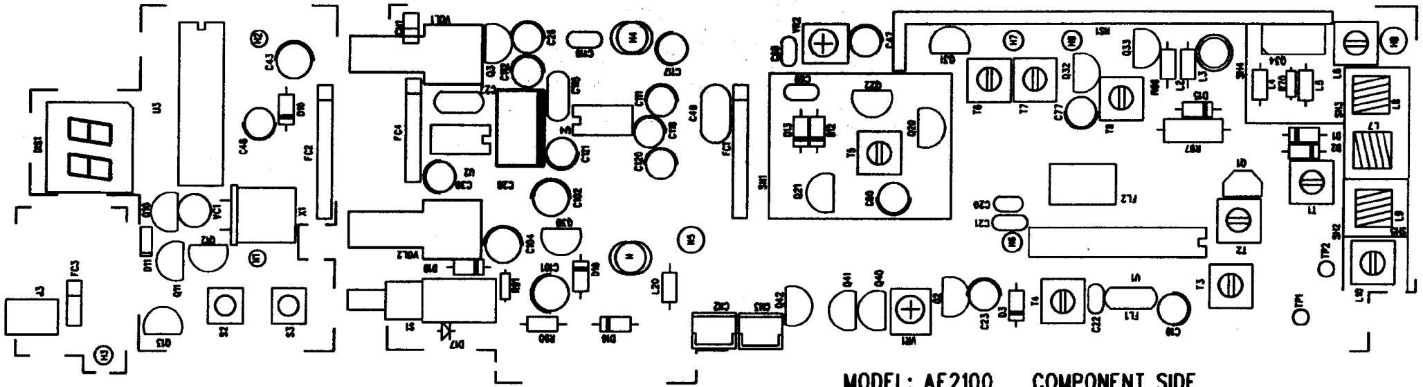
MODEL: AE2100 COMPONENT SIDE SCALE: 1:1 TELINSTRUMENT CO.,LTD.
