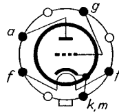
Sockelschaltschema
