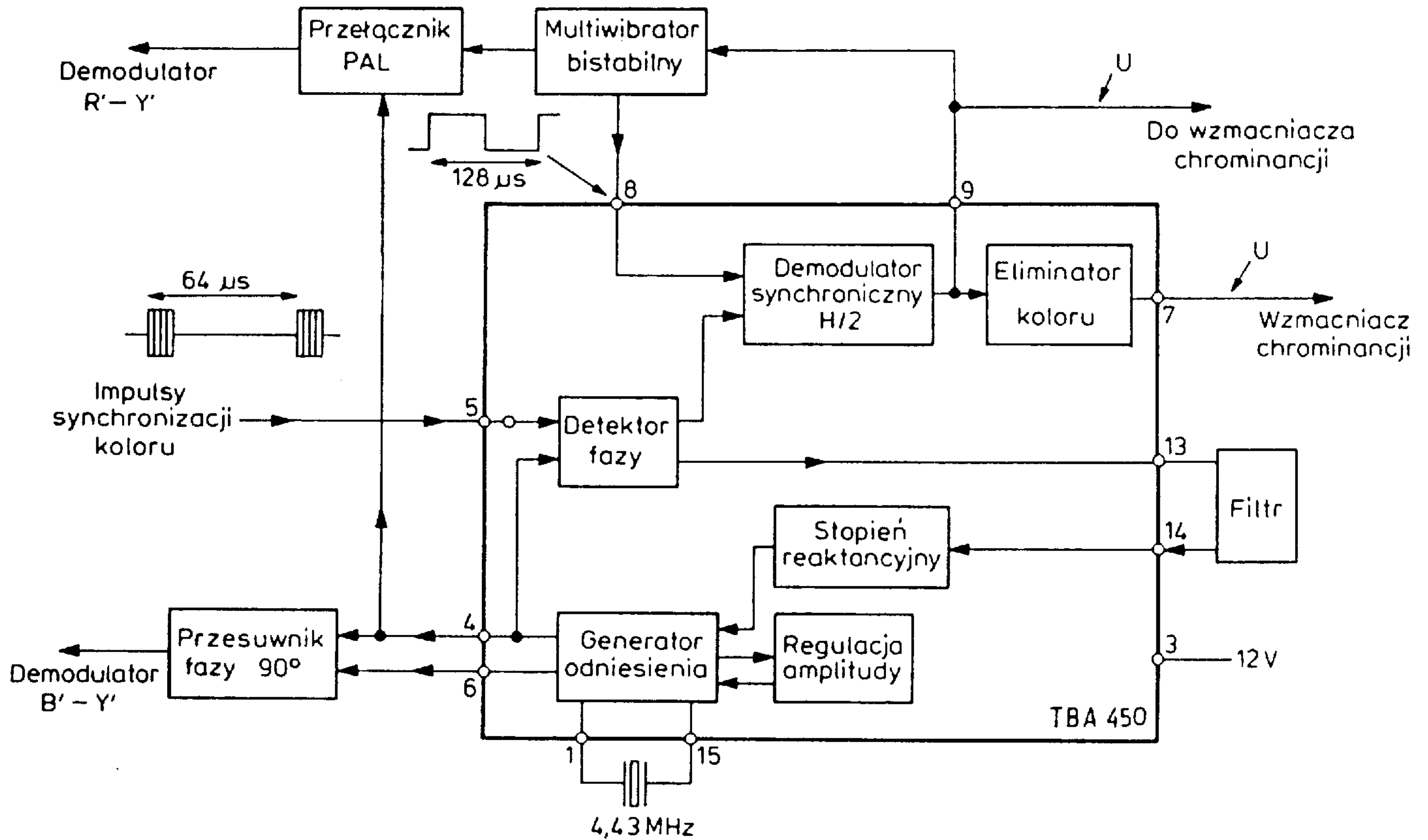
Rys. 11.4. Układ scalony TBA 450
