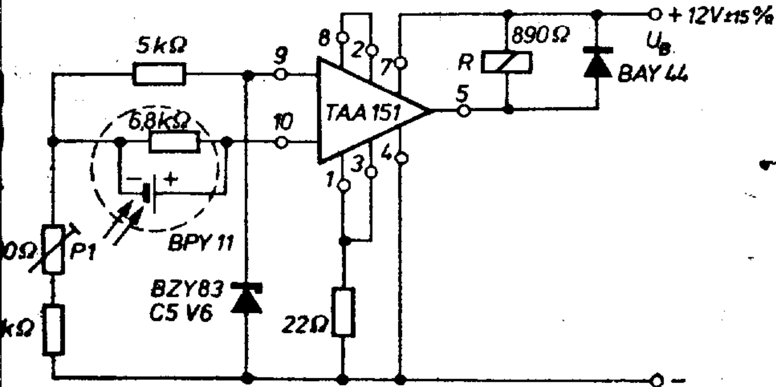
rys. 3.16. Układ sterowania przekaźnikiem R przy pomocy wzmacniacza operacyjnego TAA151 i fotoogniwa BPY11
