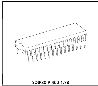
Weight : 1.99g (Typ.)
