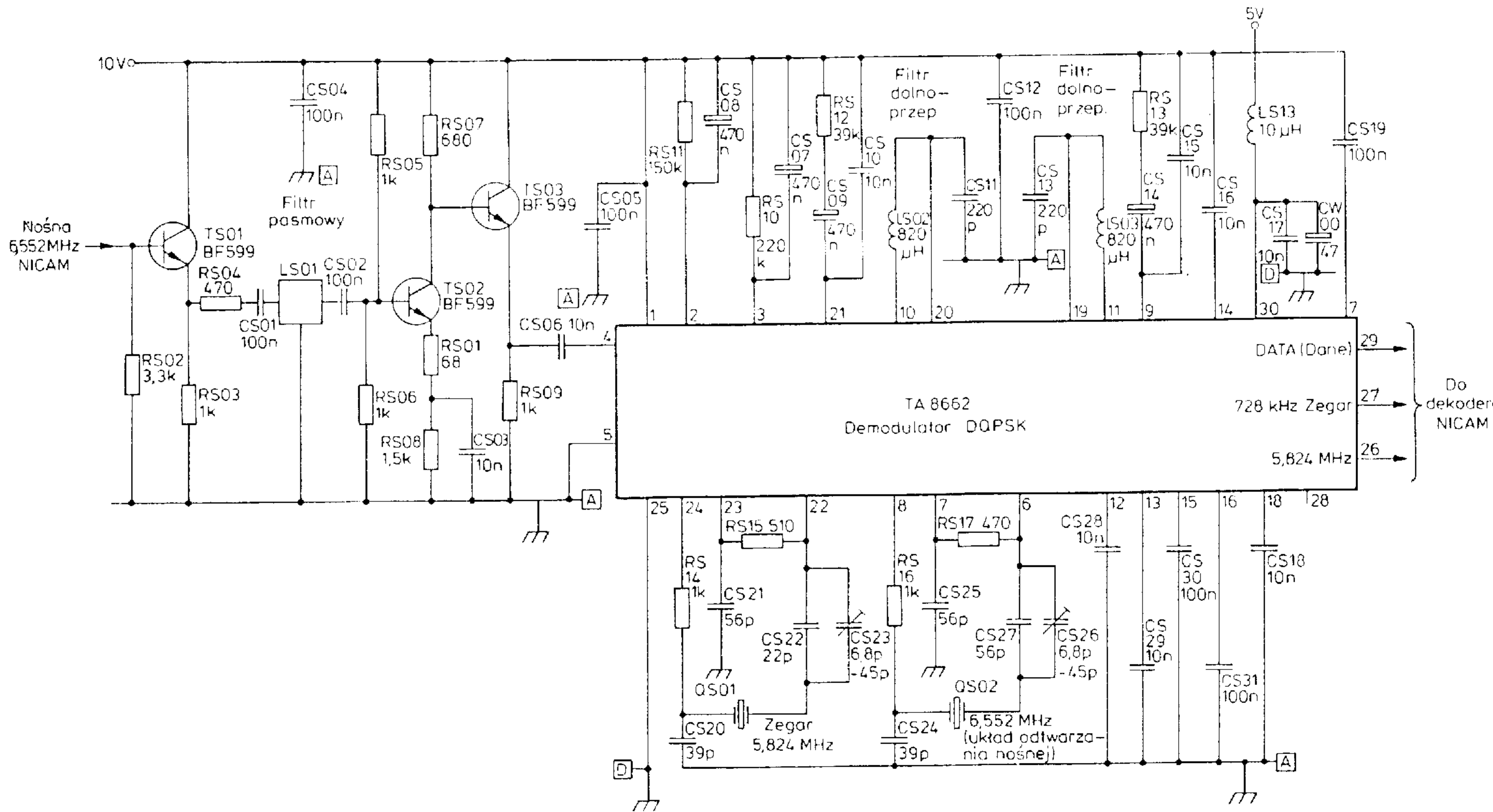
Rys. 16.13. Demodulator DQPSK z układem scalonym TA 8662 (Fergusona)
