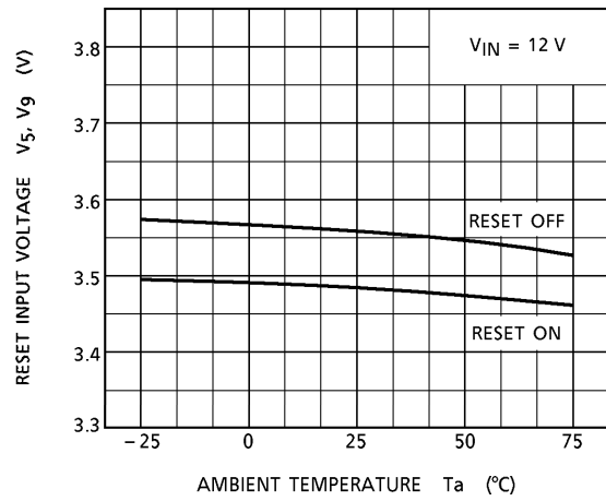
V 5 , V 9 - T a
