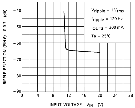
R.R.3 - V IN
