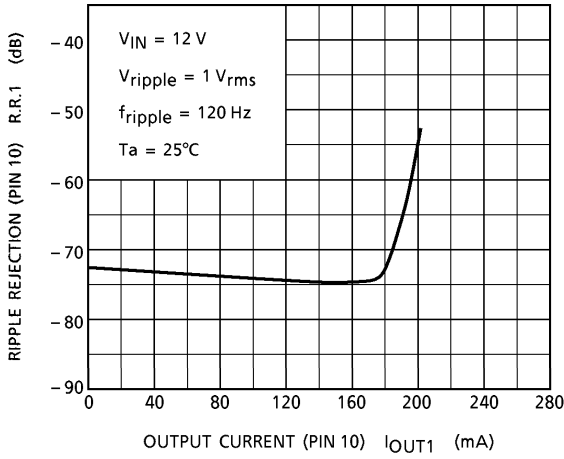
R.R.1 - I OUT1
