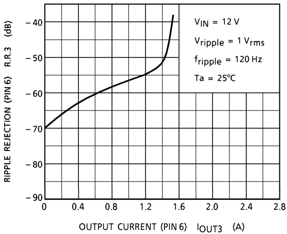
R.R.3 - I OUT3
