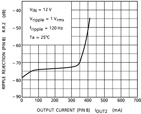
R.R.2 - I OUT2
