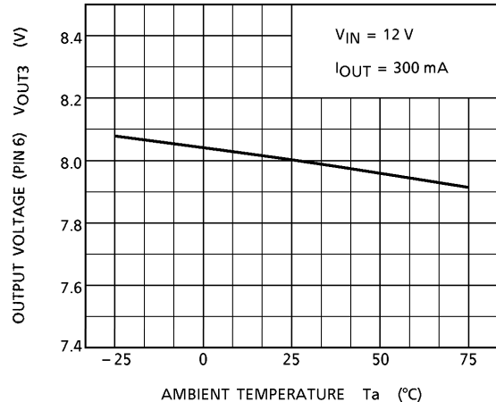
V OUT3 - T a
