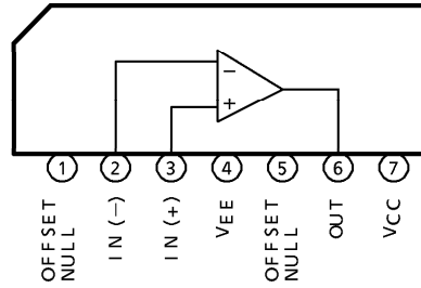
TA75071S
