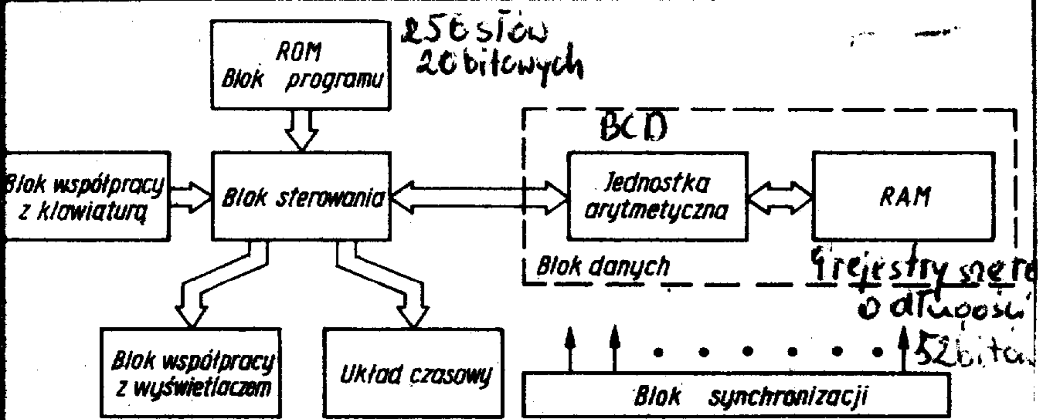
Schemat blokowy układu scalonego MC1930
