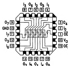
TL/F/10659-3
